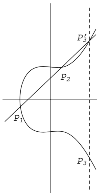
图 3: 群运算
